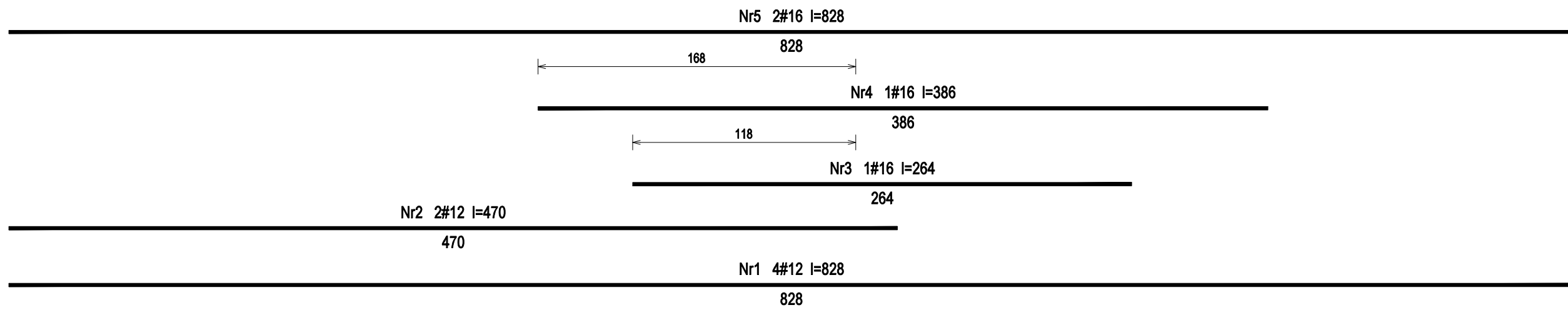
POZ.1.52 - Wykaz zbrojenia dla 1szt.
